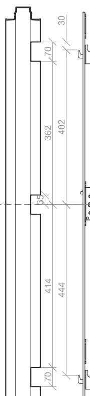
259017 y 259020 Multipuntos 1000 mm
