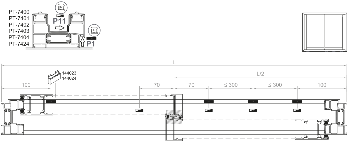
Desagües en marcos de 2 carriles
