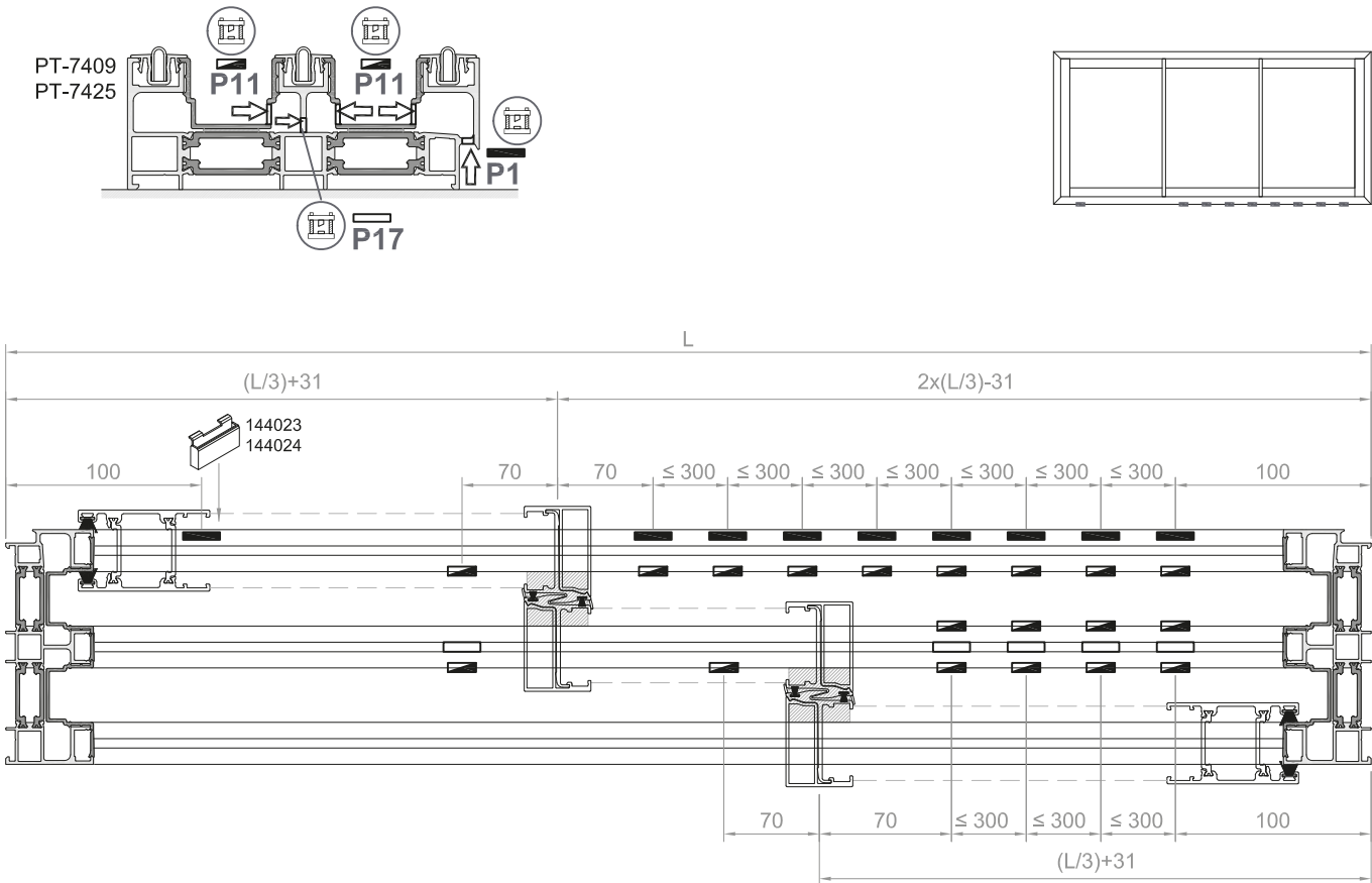
Desagües en marcos de 3 carriles
