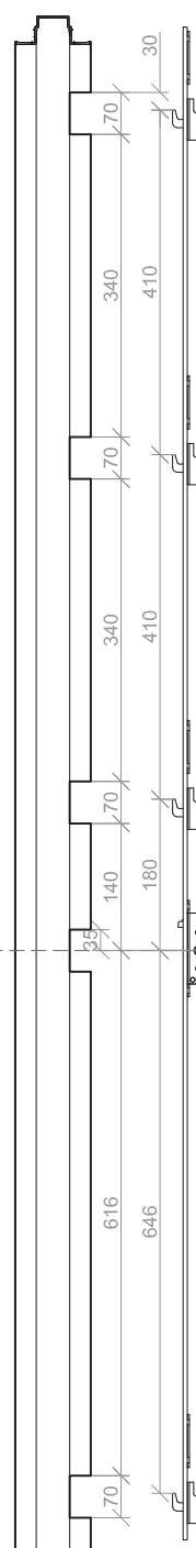
259019 y 259021 Multipunto 1800 mm
