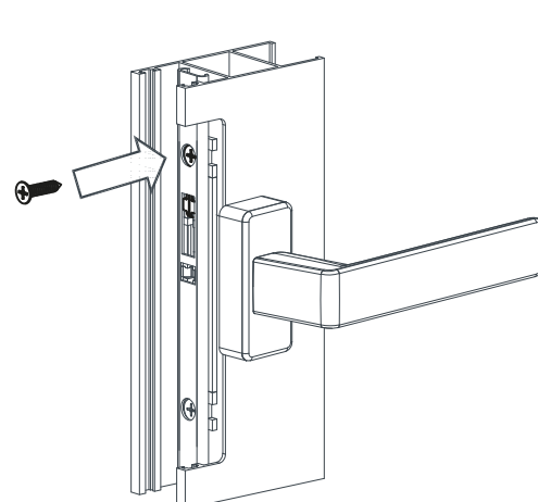
07 Introducción del tornillo para fijación de la pieza de bloqueo.
