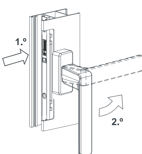
06 Introducción completa de la pieza de bloqueo de manera previa al giro de manilla.
