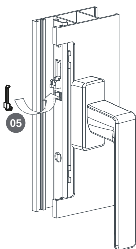
05 Introducción de la pieza de bloqueo mediante el enganche inferior.
