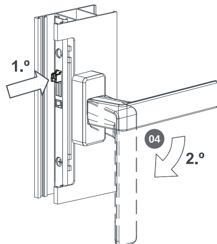
04 Presionar el anti-falsa maniobra para girar la manilla y devolverla a su posición cerrada.
