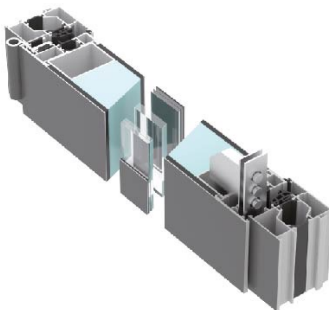
Detalle Perfilera
