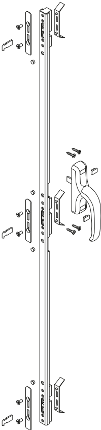
Multipunto 1000 mm
