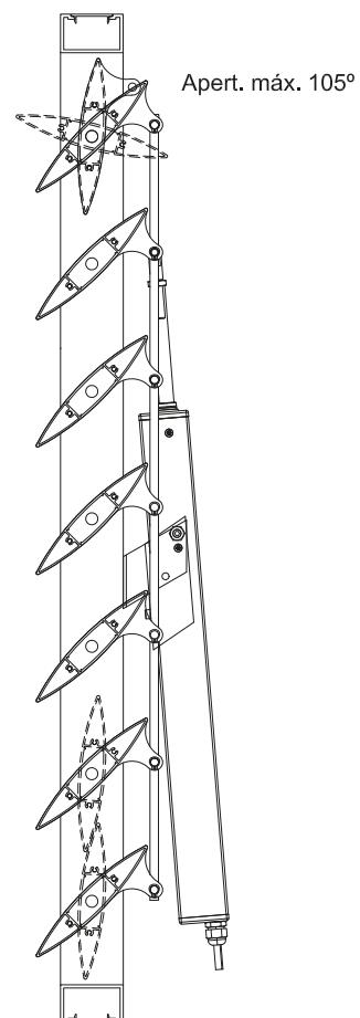
Lama de 150 mm Accionamiento motorizado
