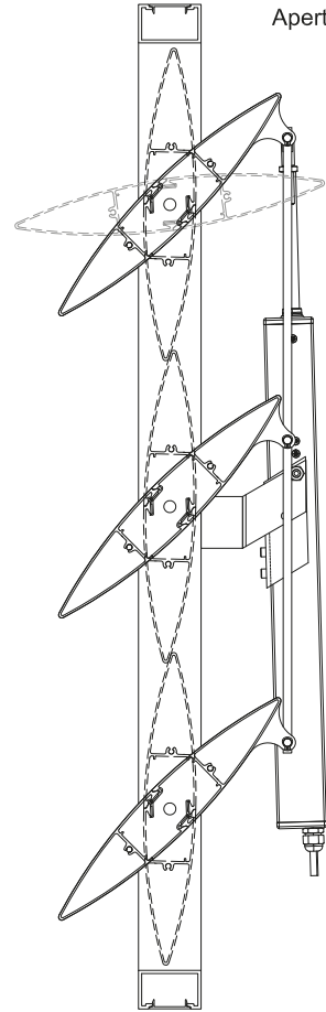
Lama de 300 mm Accionamiento motorizado
