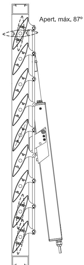
Lama de 125 mm Accionamiento motorizado
