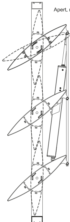
Lama de 400 mm Accionamiento motorizado
