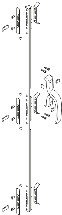
Multipunto 800 mm
